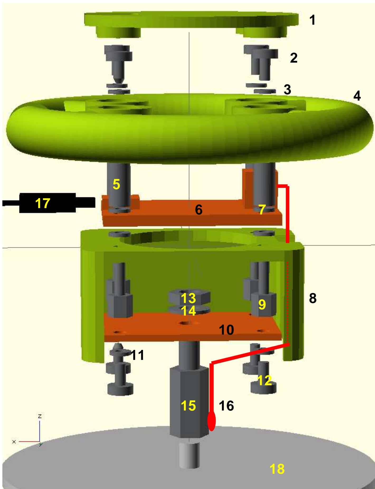
Vue éclatée de la e-poignée (voir la nomenclature)
